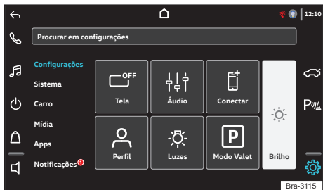
Fig. 147 Menu configurações.
