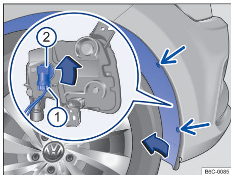
Fig. 166 Na caixa de roda dianteira: acesso à lâmpada incandescente do farol de neblina.
