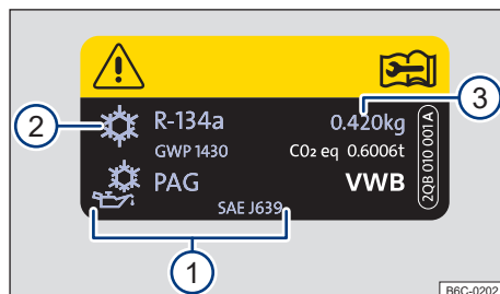
Fig. 207 Informações do ar-condicionado - motor 1.0L TSI, motor 1.4L TSI e motor 1.6L.
