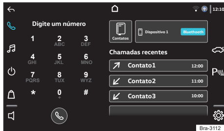
Fig. 142 Função telefone.
