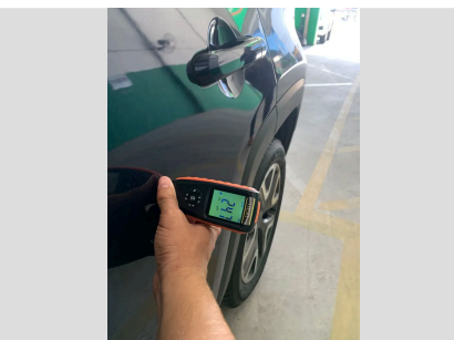
PORTA TRASEIRA LE (REPINTADO)
